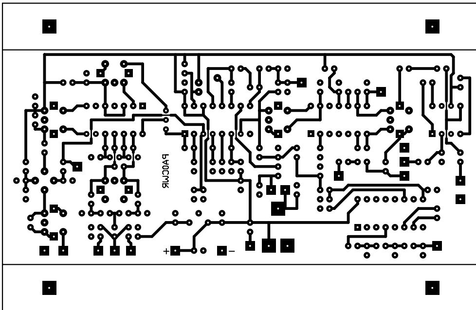
VDSRX-B Bottom Layer
